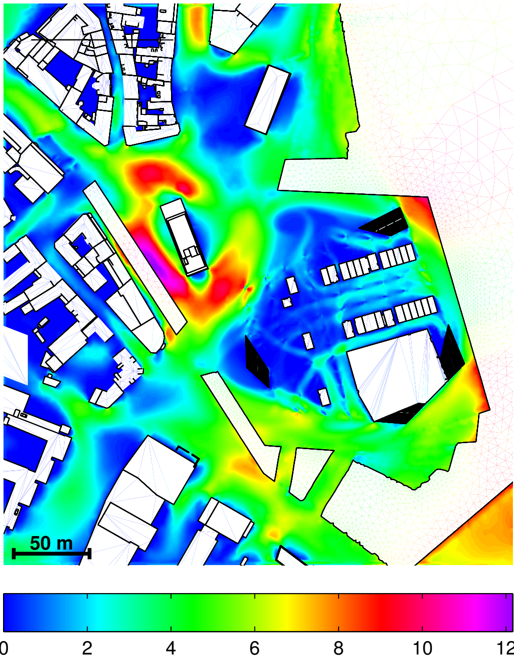
Figur 25 Konturplot af tidlig overskridelse af komfortkriteriet (formel (1)) i % på terrænniveau omkring Multimediets hus.
