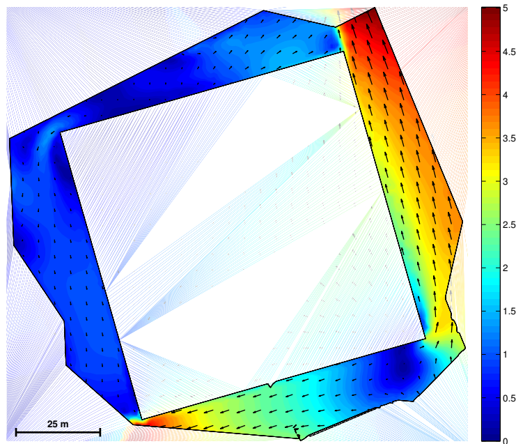
Figur 20 Vektorplot af vind fra 135^\circ i forhold til nord.
