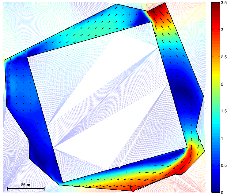
Figur 19 Vektorplot af vind fra 90^\circ i forhold til nord.
