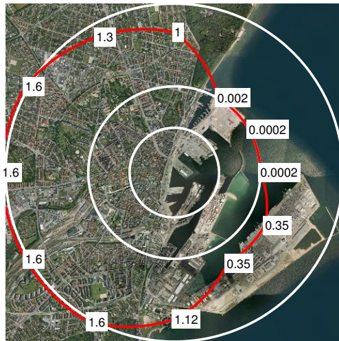
Figur 5 De lokale ruheders afhængighed af vindretning.
