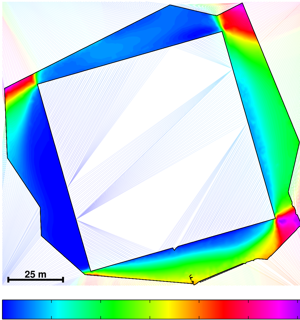
Figur 26 Konturplot af tidslig overskridelse af komfortkriteriet (formel (1)) i % på Multi-mediehusets niveau 1.
