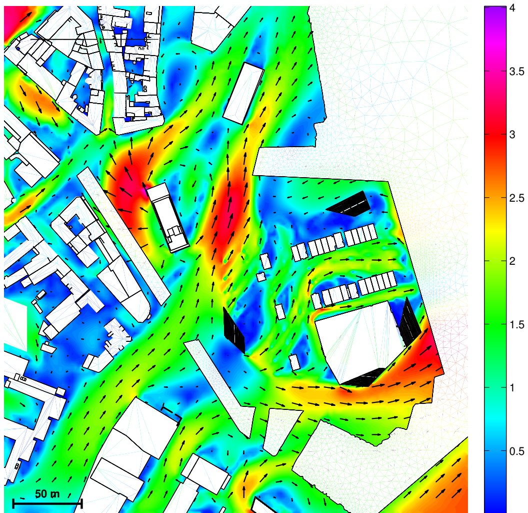
Figur 14 Vektorplot af vind fra 225° i forhold til nord.
