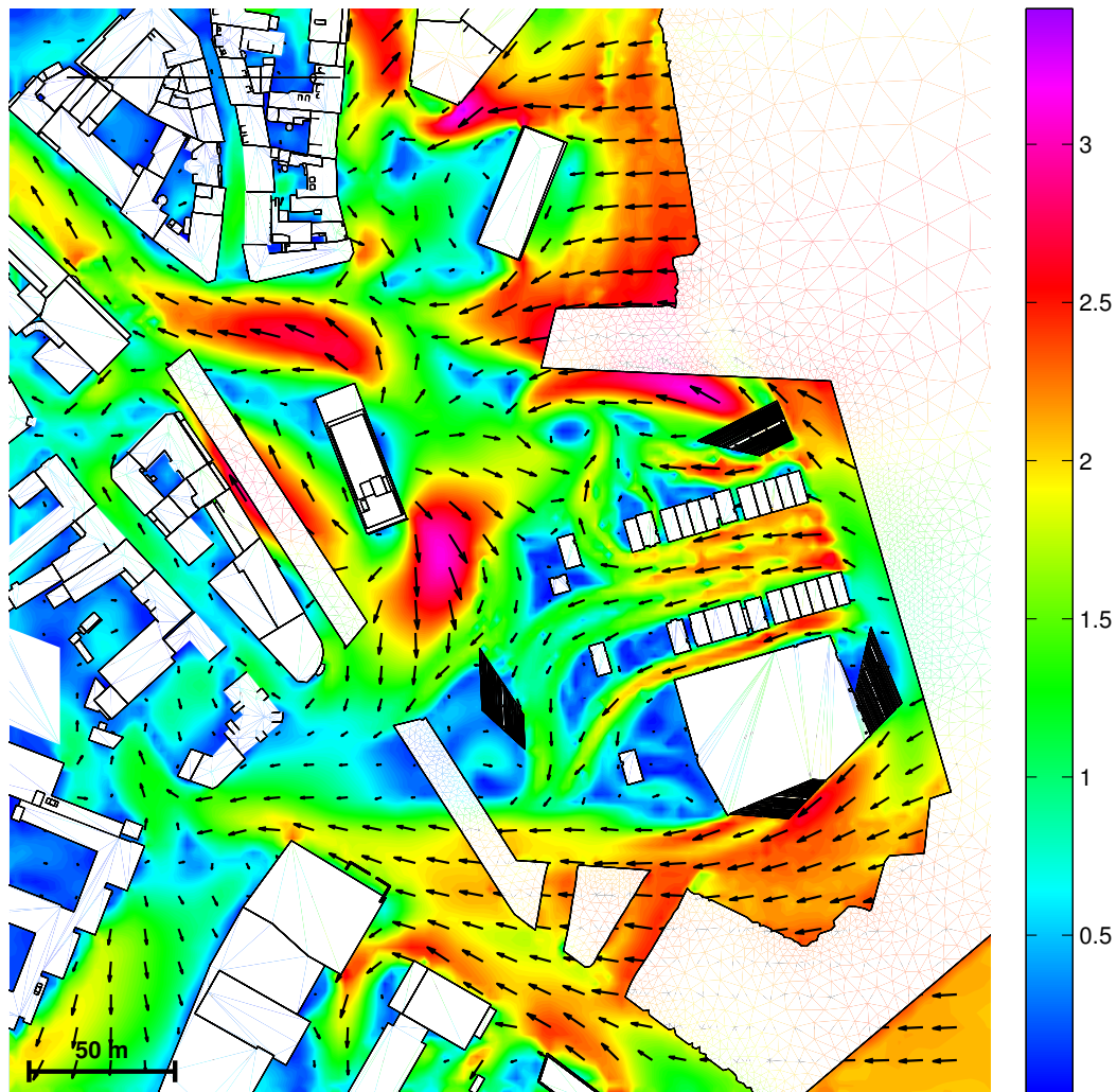
Figur 11 Vektorplot af vind fra 90° i forhold til nord.
