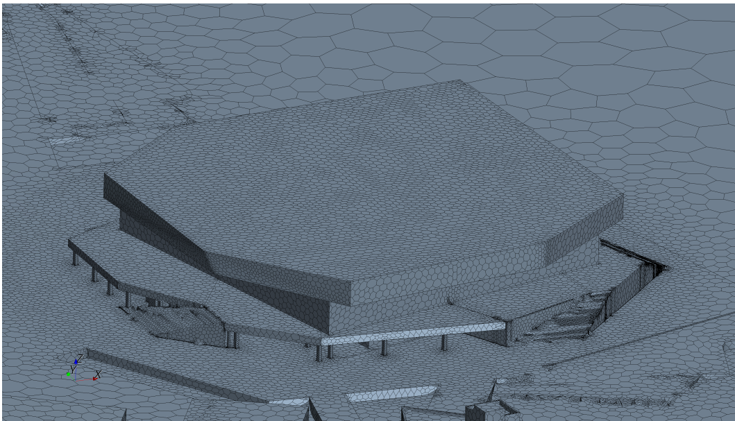
Figur 4 Illustration af beregningsnet ved Multimediahuset.
