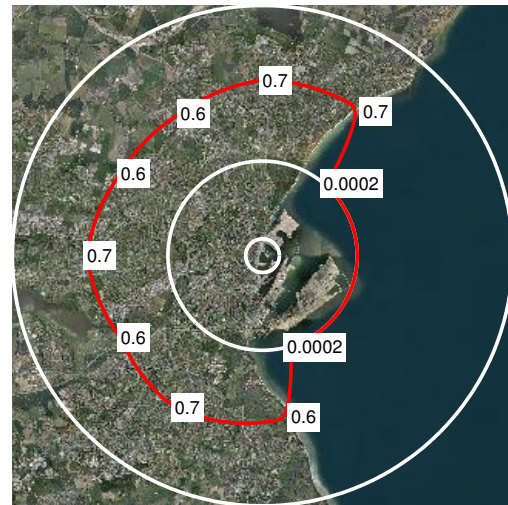
Figur 6 De regionale ruheders afhængighed af vindretning.
