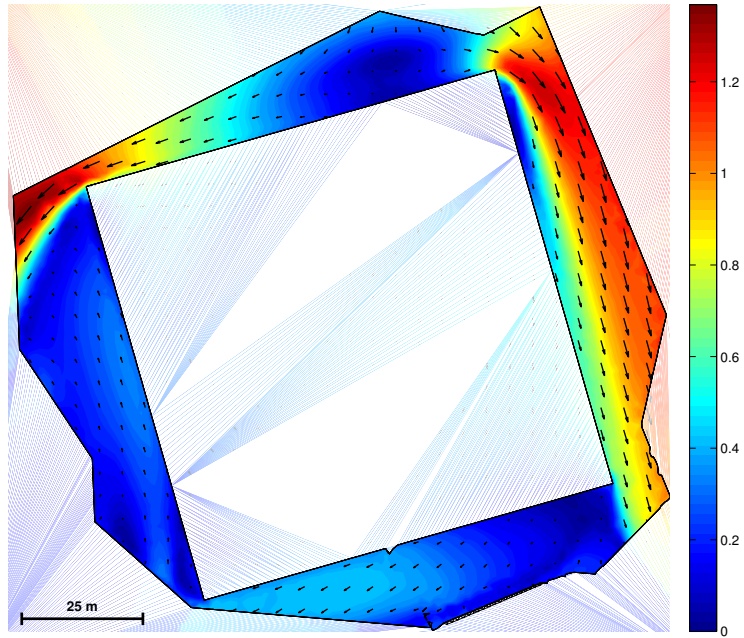
Figur 17 Vektorplot af vind fra 0^\circ i forhold til nord.
